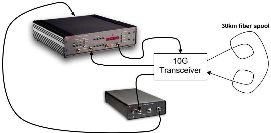
Fig. 2 Diagram with TG1B1-A and TR1C1-A
